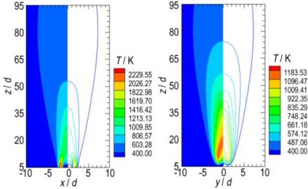
图9 5#点火具燃烧场x-z和y-z截面温度分布云图
