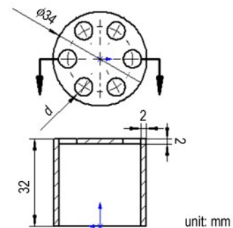
图1 底排点火具示意图
