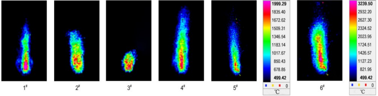
图 6 1 # ~6 # 点火具火焰红外热像图
