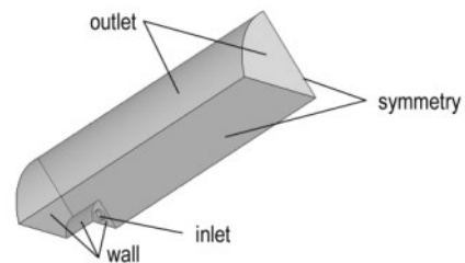
图8 计算域和边界条件
