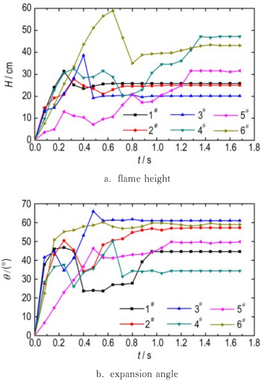
图4 I 类型点火具燃烧火焰高度和射流扩张角随时间的变化曲线
