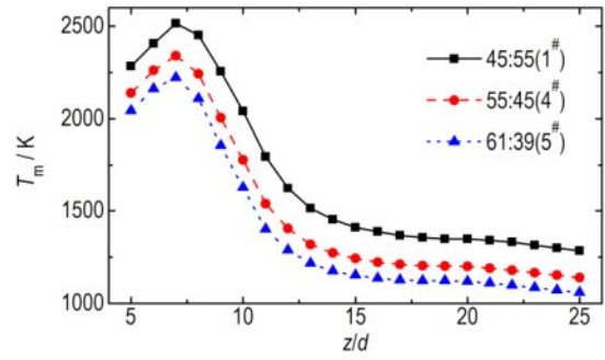
图11 孔径为6.5mm的燃烧场x-z截面纵向最高火焰温度分布
