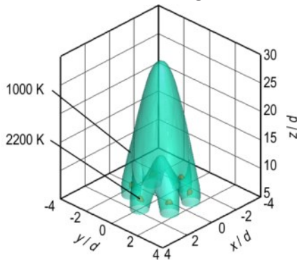
图10 5#点火具燃烧场三维温度等值面
